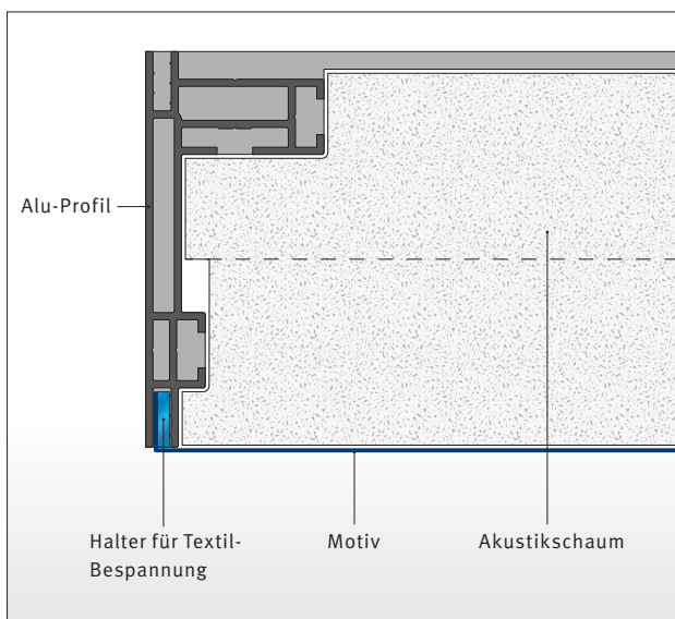
Akustik-Decken-Element SB 100
