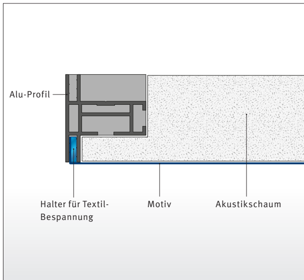
Akustik-Decken-Element FF DUO 50
