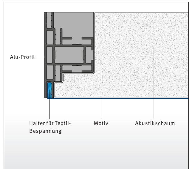
Akustik-Decken-Element FF DUO 80
